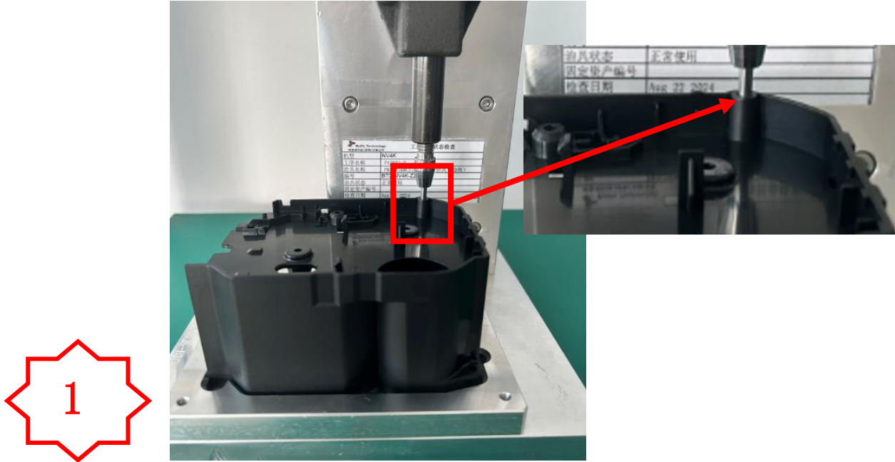
一，将 PA3861-2 组件放入治具装上 MC2226 后进行压合。
