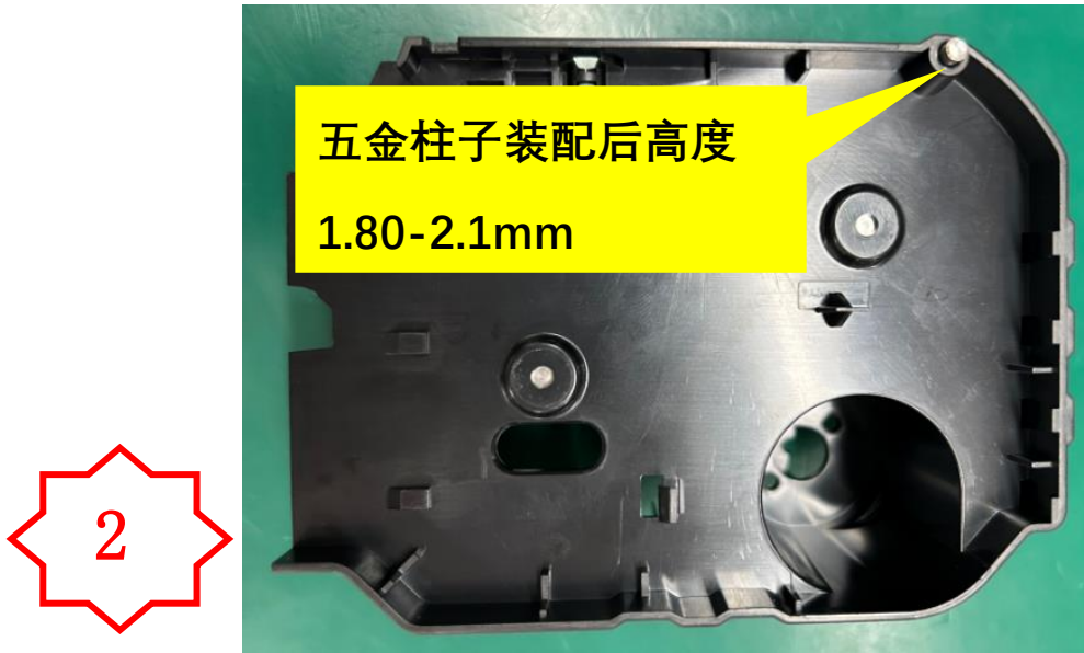
二，检查压合到位后五金柱子高度为：1.80-2.10mm。
