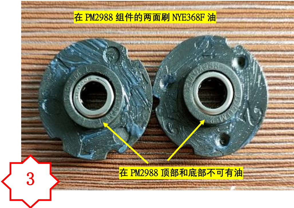
图三，检查刷好的组件两面都需要有油
