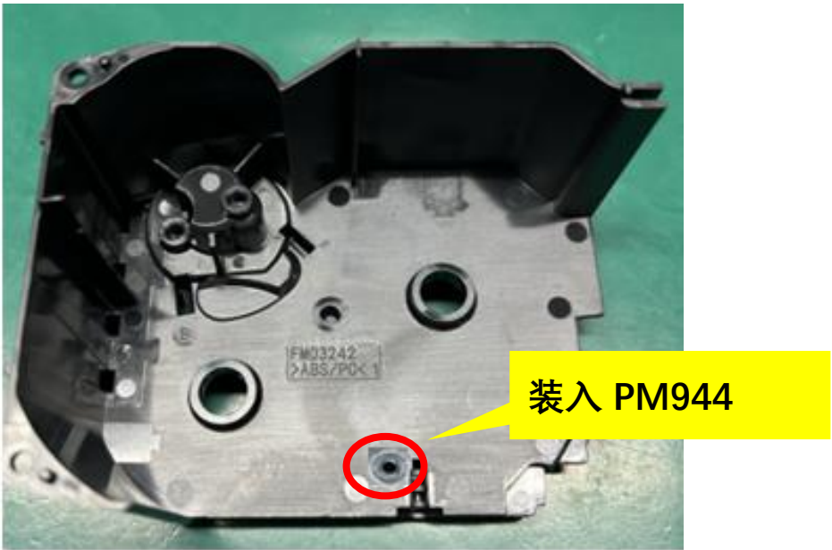
二, 将 PM944 装入红色圈圈位置, 注意装配到位 。
