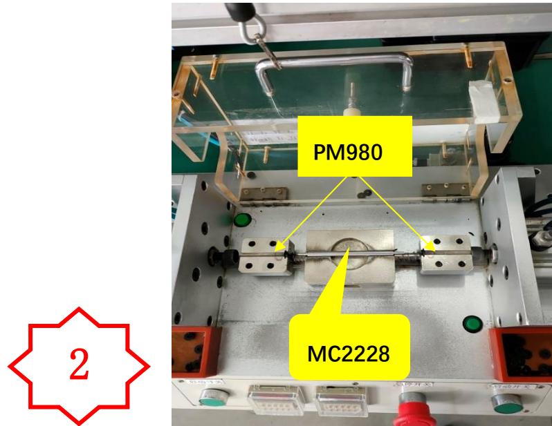
图二，先将 PM980*2 和 MC2228 放到治具中,关闭治具保护罩进行压合
