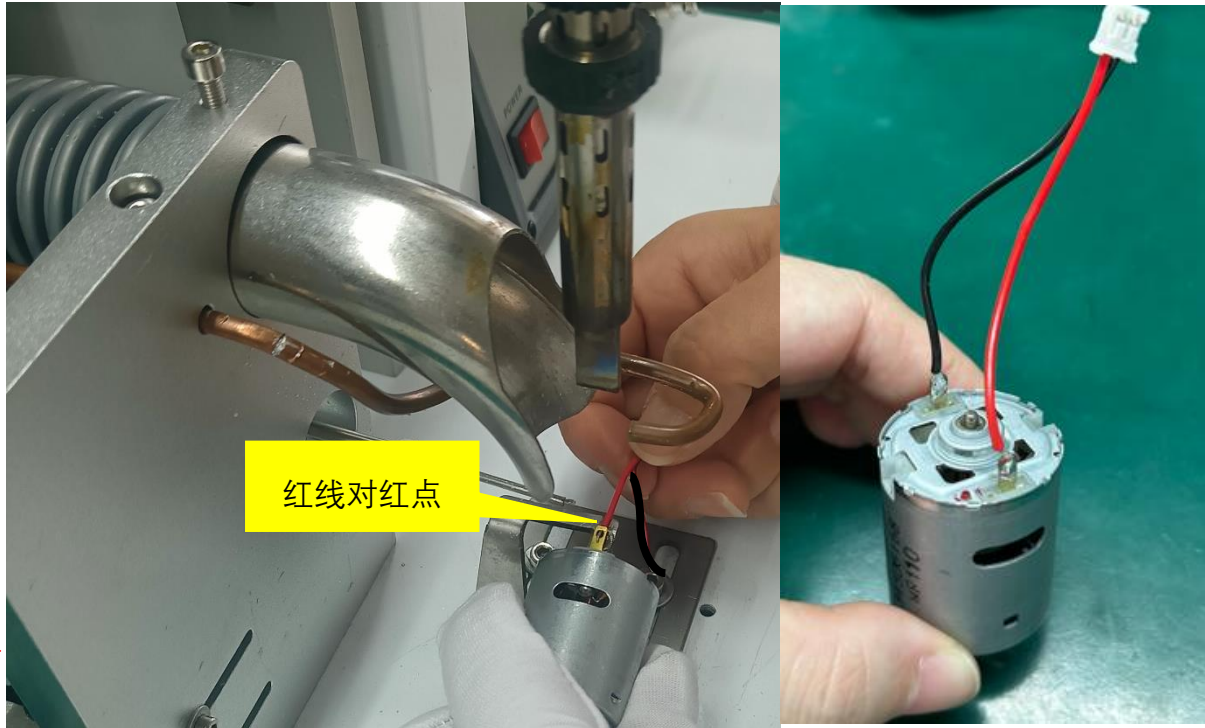
图 1. 将 CN410 的 红线 对准 PA3863-1-MR110 马达红点焊接，注意 2 个端子焊锡需饱满。
